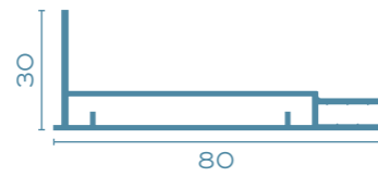
LED-ES-100-SKY Art.-Nr.: 130089
