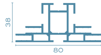
BASIC-DS-150-M.-NUT
