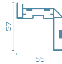
LED-ES-57-AURA Art.-Nr.: 130170
