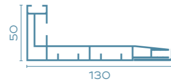
LED-STREBE Art.-Nr.: 130181
